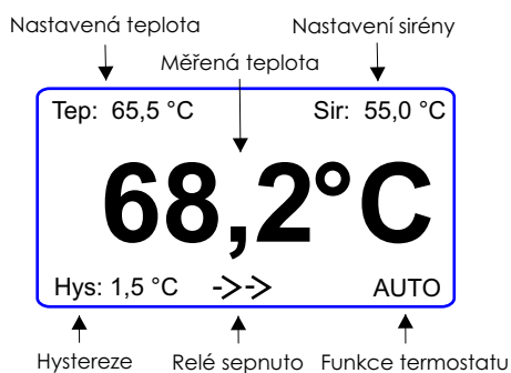
zobrazení displeje u DP 2
