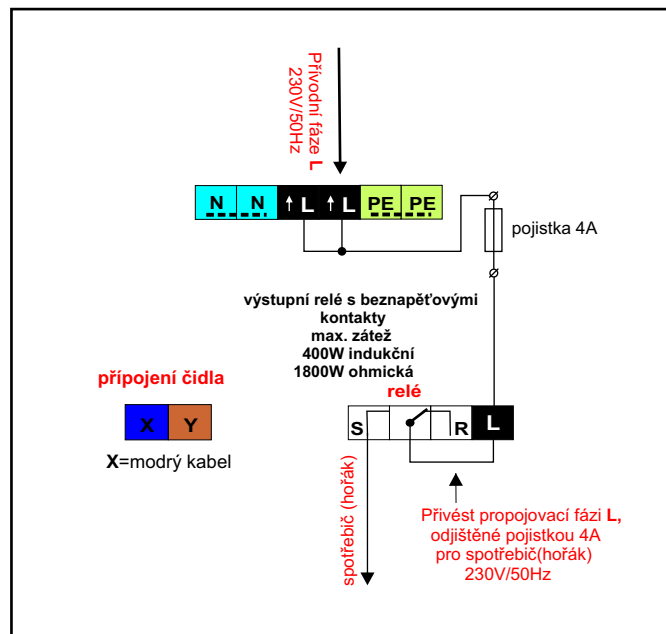
zobrazení svorkovnic - shodné pro oba typy
